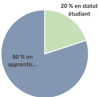
Taux d'apprentissage
