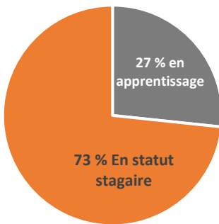
Taux apprentissage
